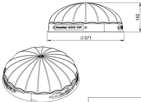
DÔME EN CRISTAL
